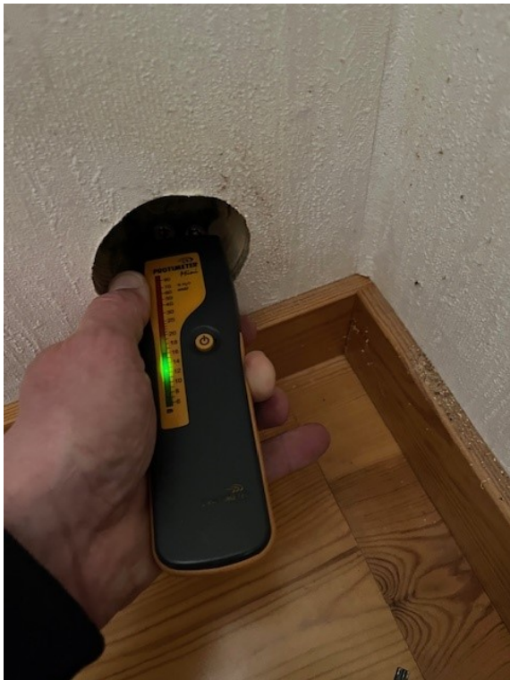
Fuktmätning i ytterväggssyll/bottenregel i kök.
