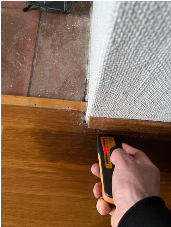
Fuktmätning i parkettgolv i gillestugan.
