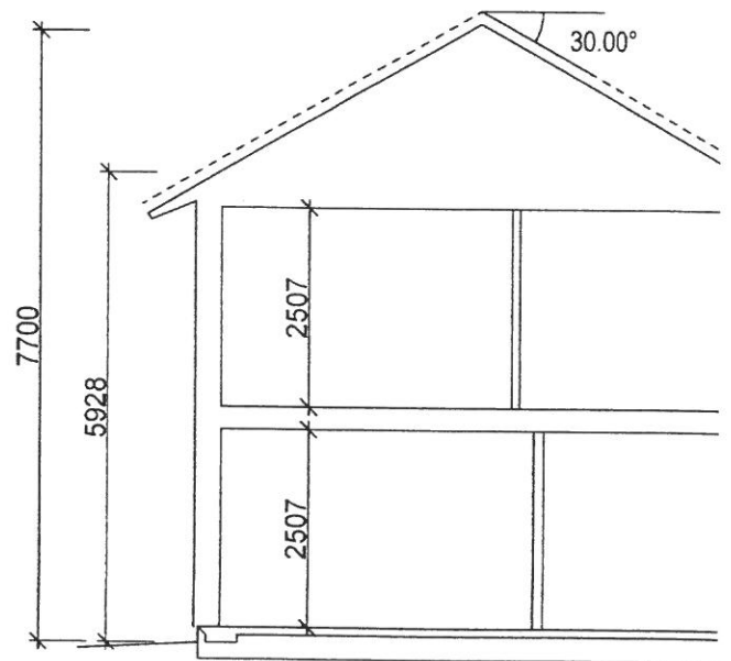
SEKTION A-A
