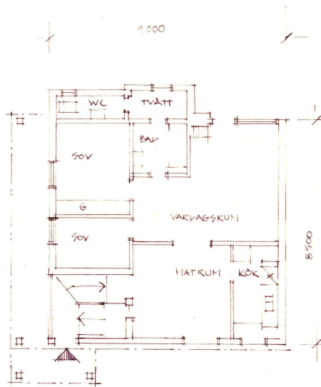
VÄNINGPLAN
