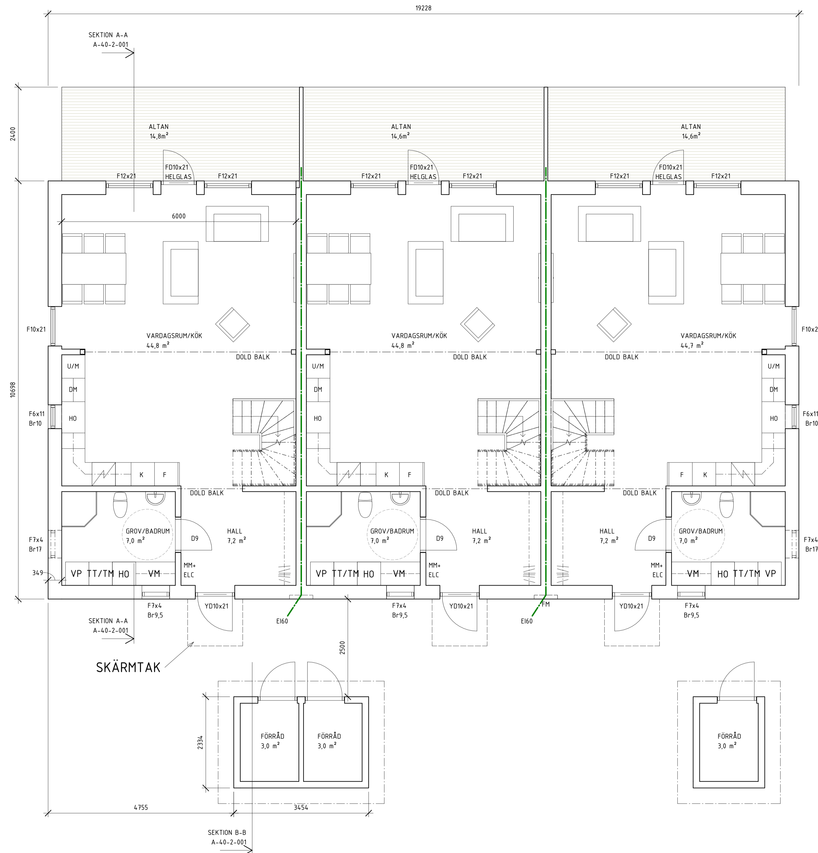
BOTTENPLAN 1 : 50
