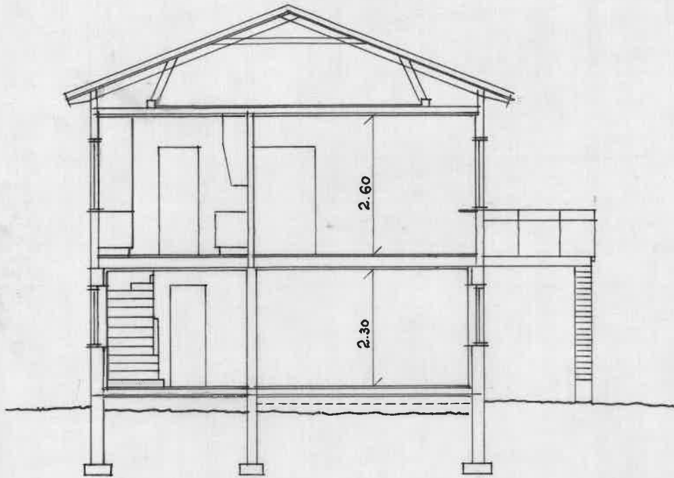
SEKTION
