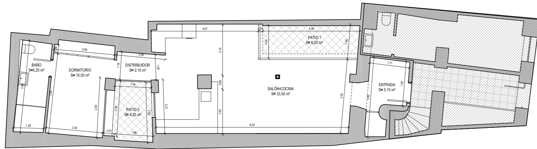
VIVIENDA A acotada
