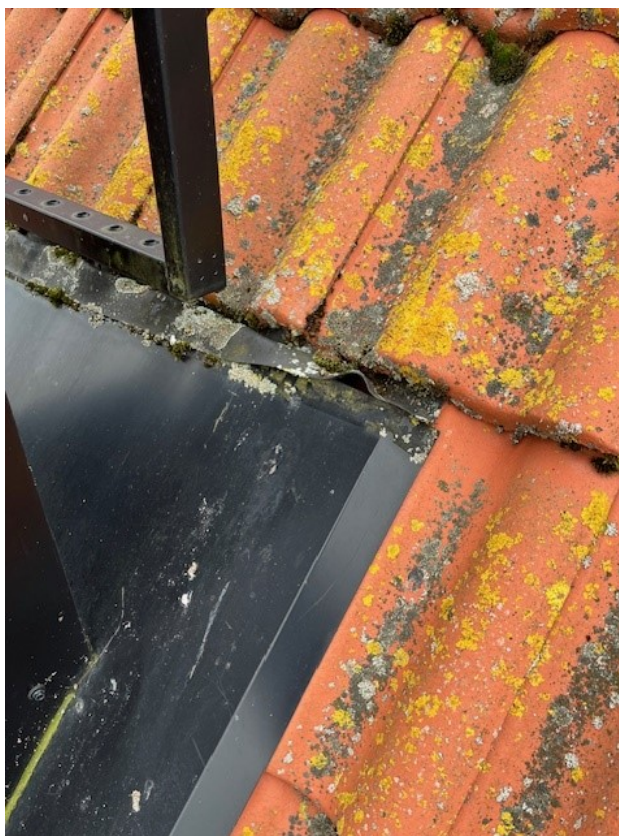
Tätning över skorstenens genomföring som släppt något från sin infästning.
