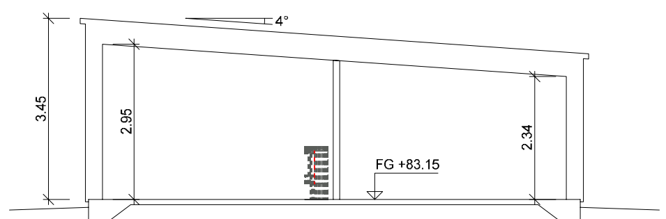
SEKTION A-A
